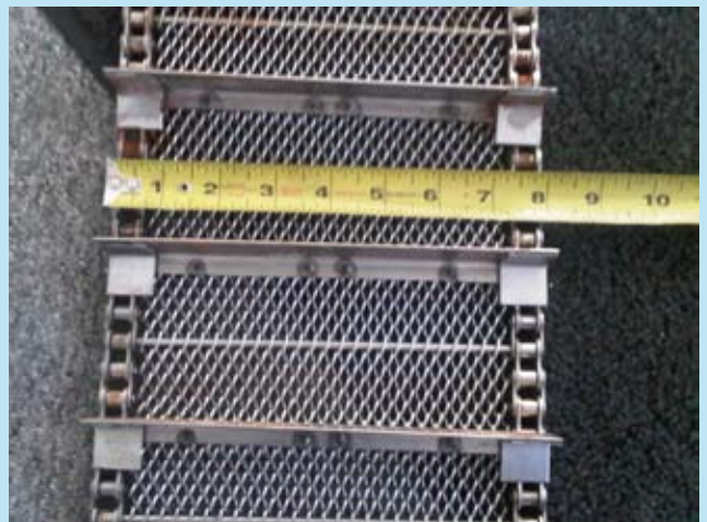
Treillis avec ferrantes soudées sur treillis
