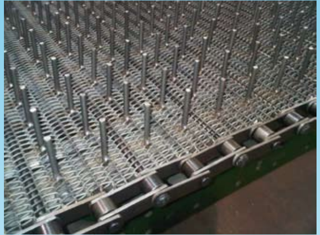
Attachements inox soudés sur treillis
